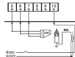
紫外探头检测
