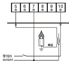
单电极检测
